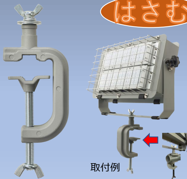
MKO用クランプ 型番：MKO-C
